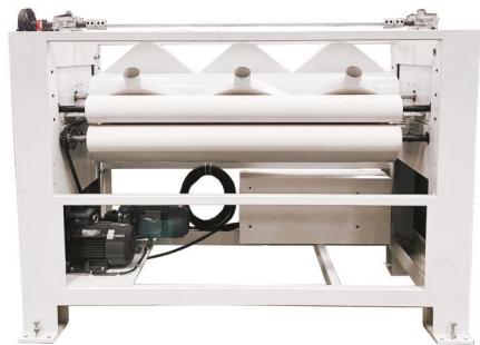
TCC-A 毛扫辊双面除尘机 TCC-A Double side roller brush dust cleaner
