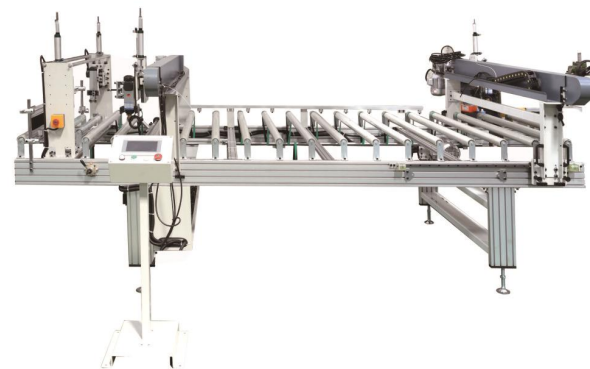
TSS-R 磨边倒角机 TSS-R panel edger
